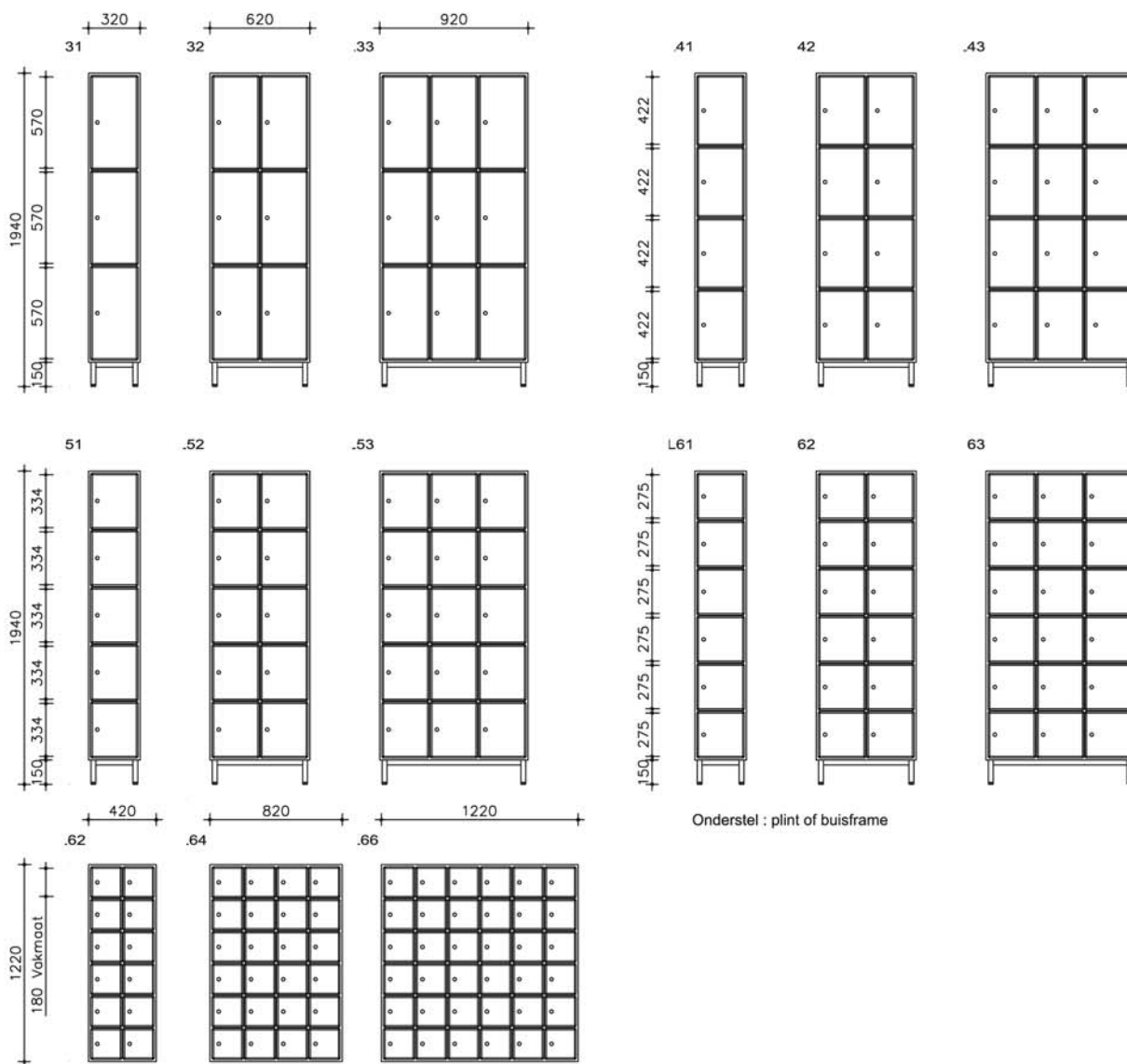
Kasten wandmontage
